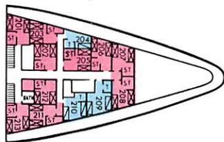
HAUPT-DECK
