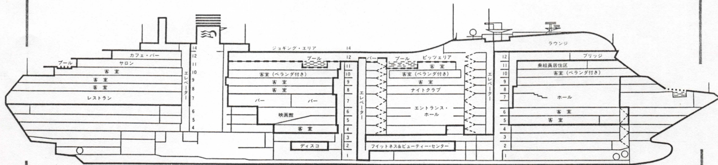
クラウン・プリンセスの側面／船内配置図
