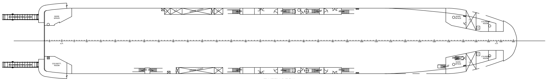
TWEEN DECK
