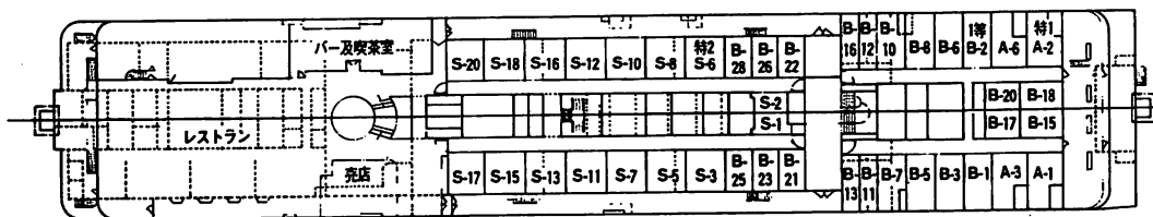
B-DECK サロン甲板
